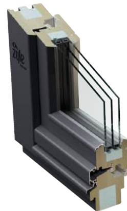
Passivhaus Wood Clad
